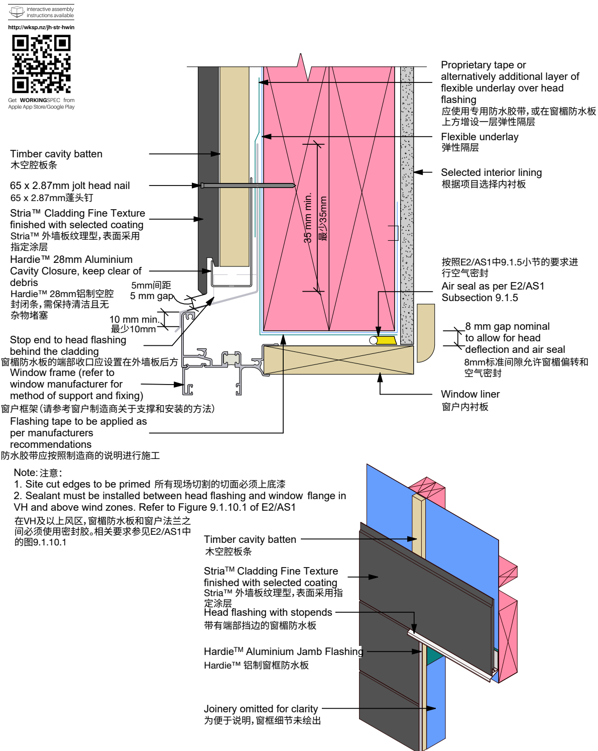
图20：外墙板覆盖着防水板的窗楣
