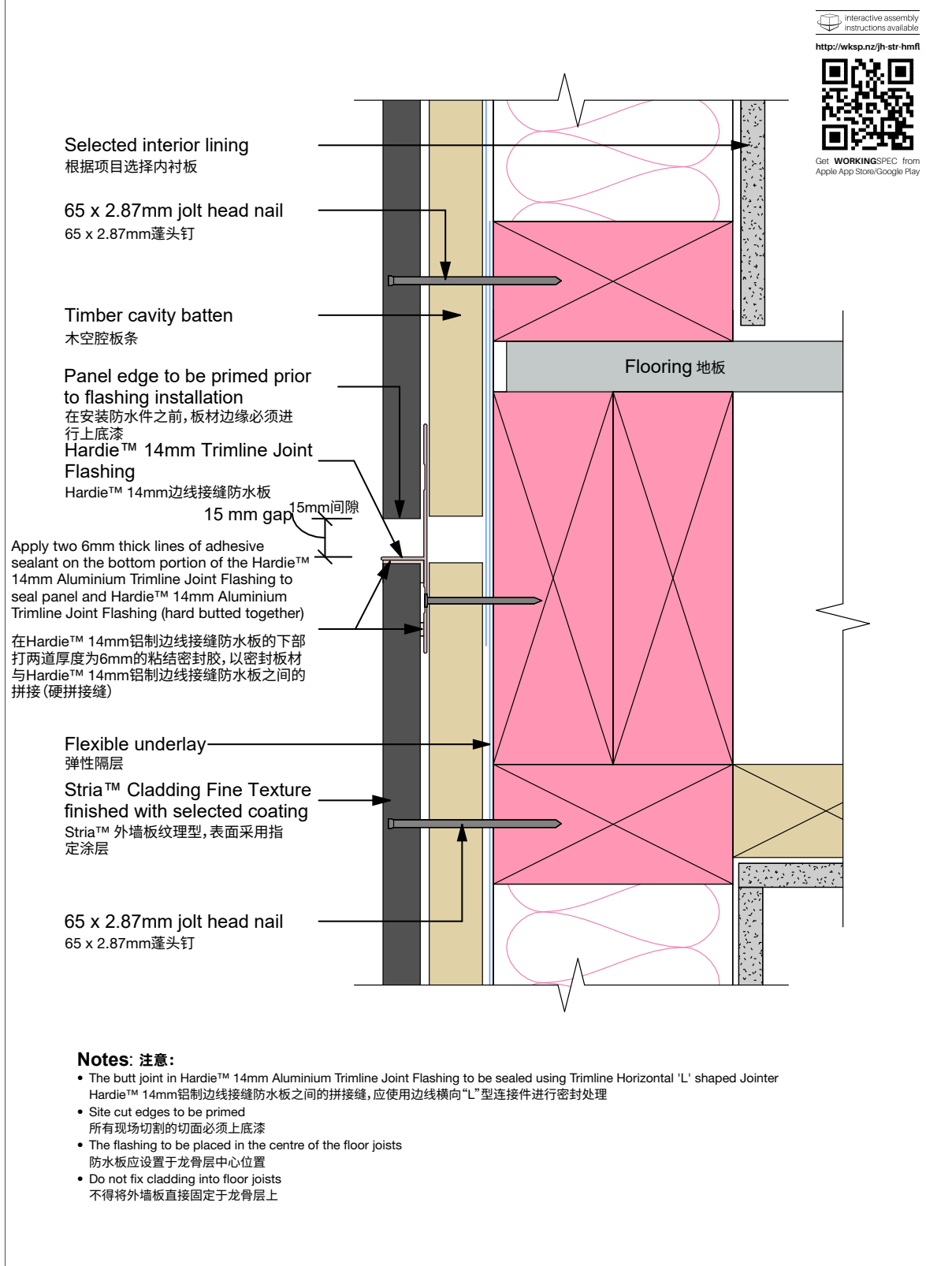
图28：龙骨层的横向接缝连接
