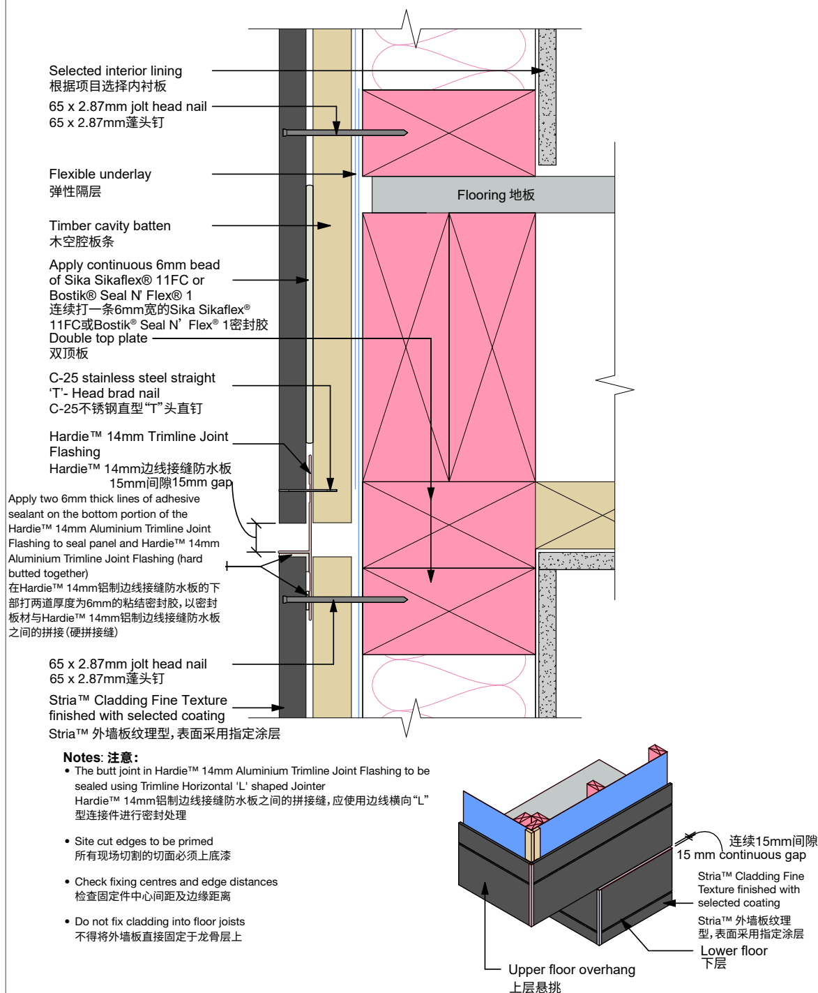
图29：龙骨层下面的边线接缝防水板连接
