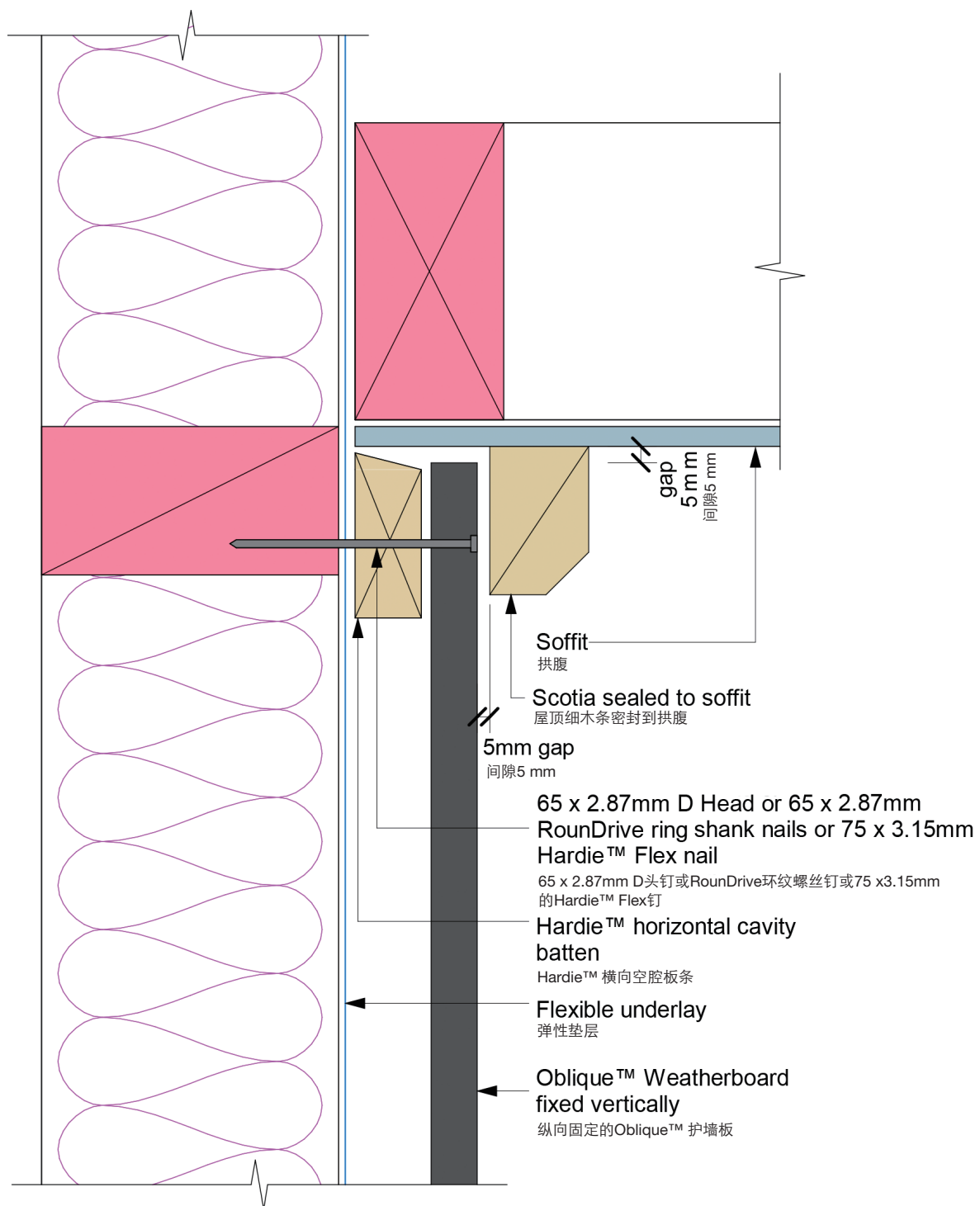
图14：拱腹顶部通风详图
