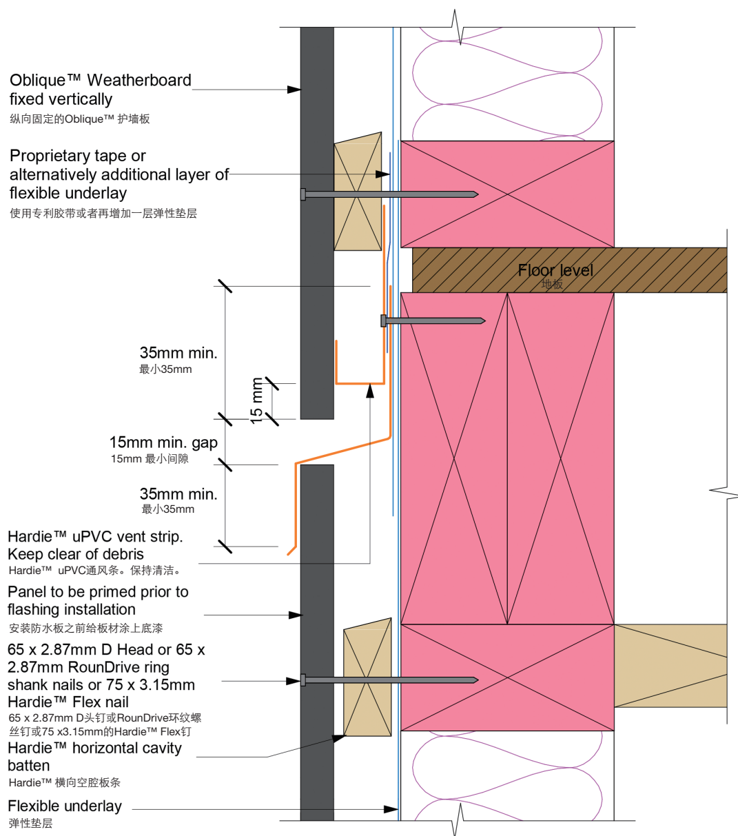
图27：地板层排水防水接缝
